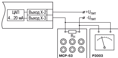
Рисунок 8.8 – Подключение ВУ1 типа У ( R_n=500 \text{ Ом} )
