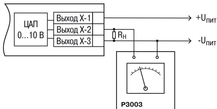
Рисунок 8.7 – Подключение ВУ1 типа И ( R_n=500 \text{ Ом} )
