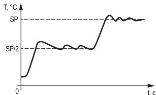
Рисунок 7.13 – Колебания в системе «нагреватель»
