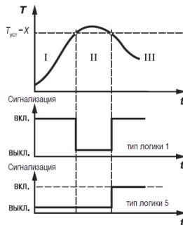
Рисунок 7.14 – Срабатывание сигнализации в системе нагрева
